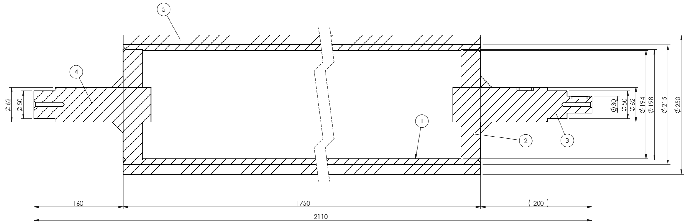
SEZIONE A-A
